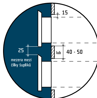
konstrukce korpusu (mm)
