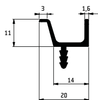
výkres k úchytkám E37, E38 (mm)
