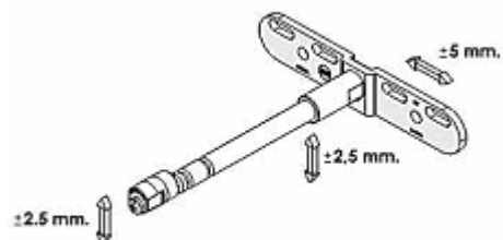
skrytá policová konsola 350 mm zinek / trn T/
