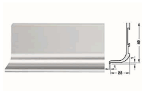
126.37.000 Zapuštěná úchytky alu.ststc.2500mm
