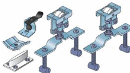
S 40H -Sada kování do 40 kg /14C0S40H/
