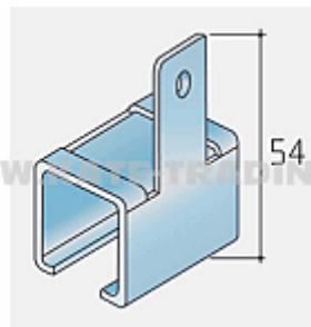
Boční úchyt na lištu S80 /14C0S4UB/
