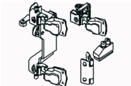
Sada kování S40SD (levá / pravá) /15C0S4SD/
