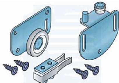
Sada kování S 37 pro posuvné skříňové dveře /13C0S37/
