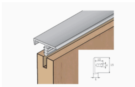
Narážecí hrana úchytná lišta S01 /1ND1NH01/ 1bm
