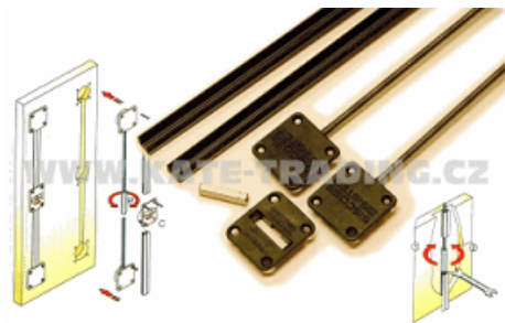
Výztuha dveří - napínák pro křídlové dveře
