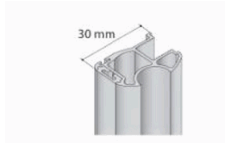
Profil boční S18 DOPRODEJ 2.70m stříbrný elox+krycí profil /17D1MS1827/
