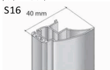
Profil boční S16 2.70m stříbrný elox+krycí profil/17D1MS1627/
