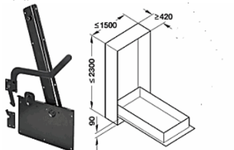
271.95.203 Kování pro sklopnou postel podélná montáž
