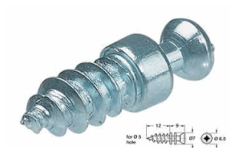
Exc-M20 Spojovací táhlo pro otvor 5 mm
